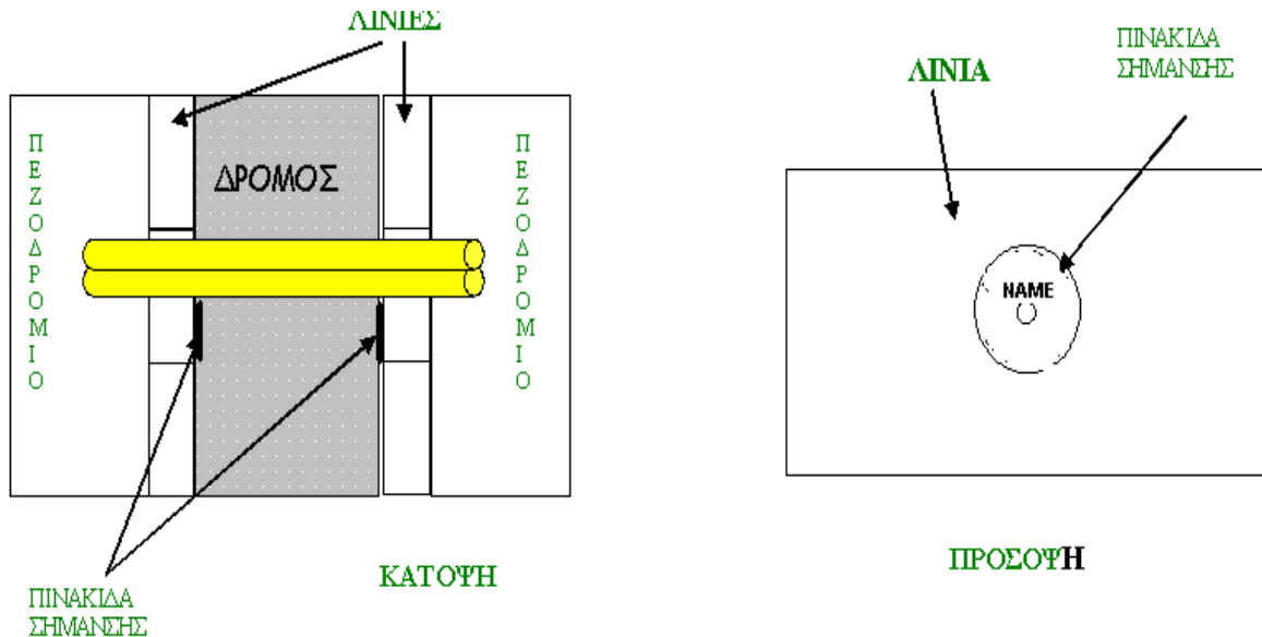
Σχέδιο 1 : Σήμανση άκρων διασταυρώσεων σωληνώσεων
